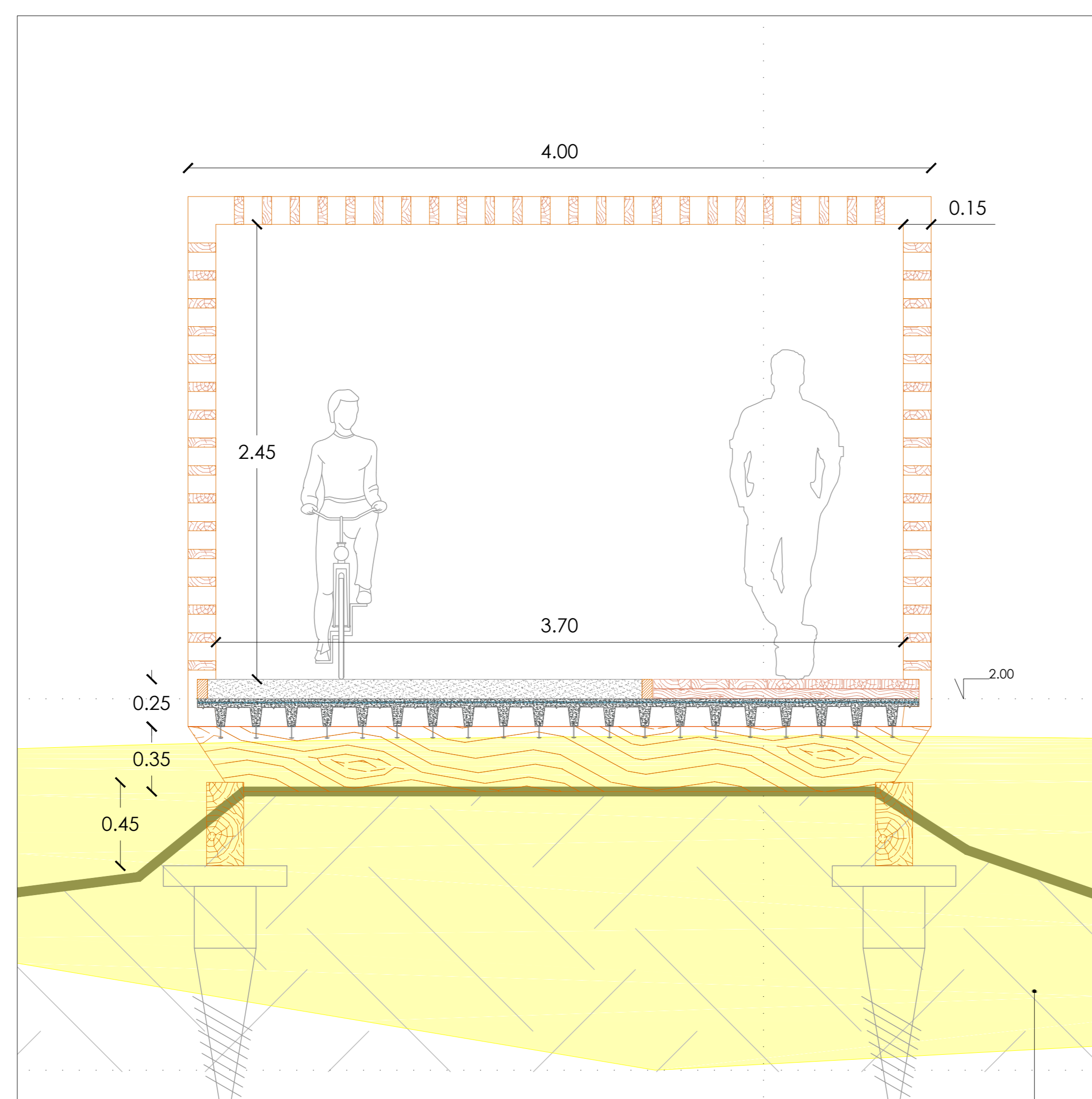
dettaglio 1 caso 1° la struttura del nuovo percorso ciclopedonale intercetta l'attuale percorso esistente, soggetto a totale demolizione, e poggia su ferrapieno nell'ambito della "depressione lagunale in seconda linea" formata in conseguenza della demolizione dell'attuale tracciato viario
